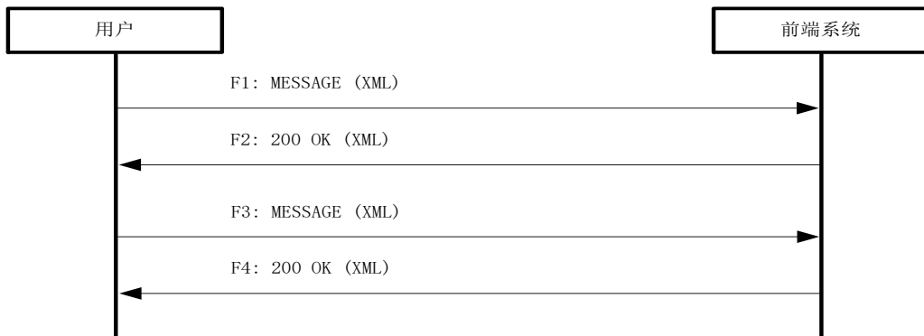
图C.15 图像参数获取及配置流程
