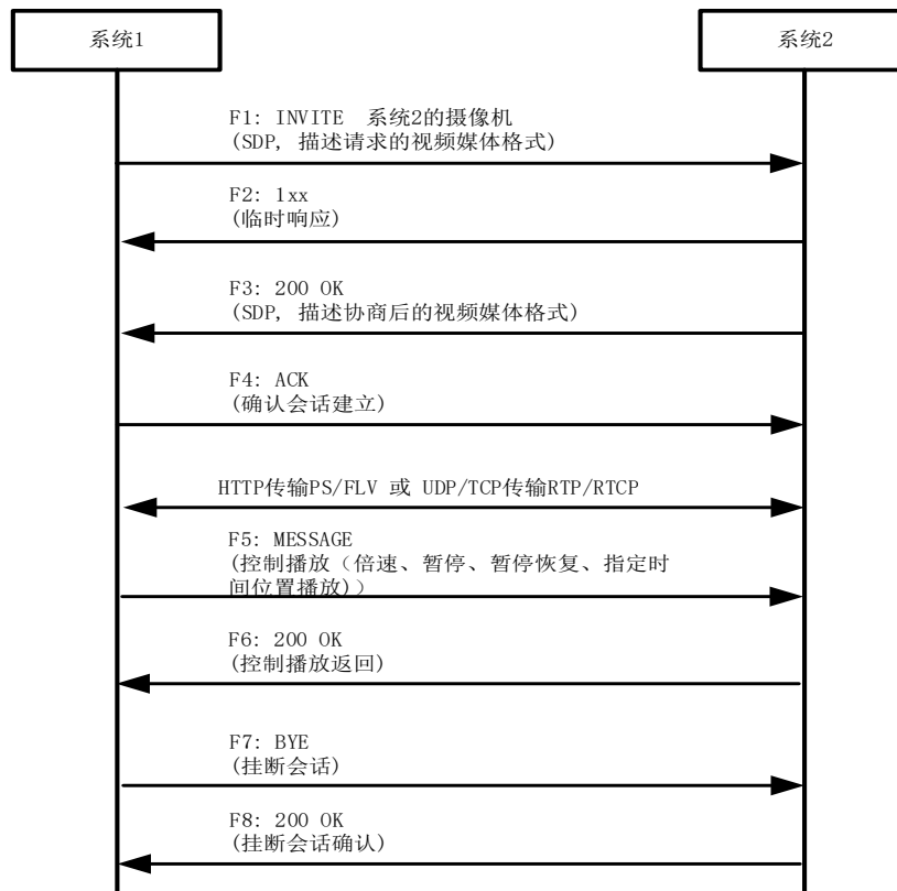
图A.14 录像回放接口流程
