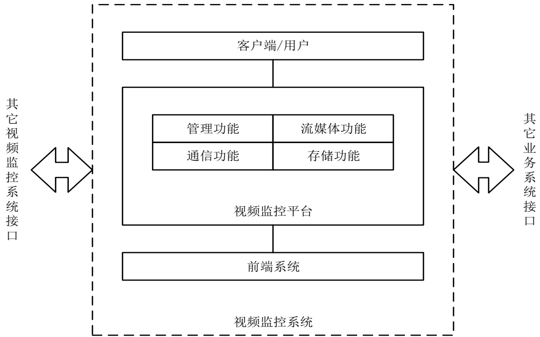
图1 视频监控系统组成示意图
