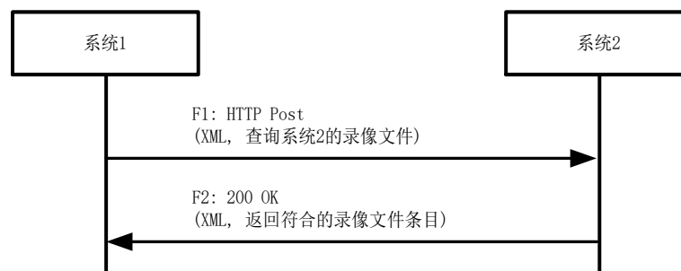
图A.5 录像检索接口流程
