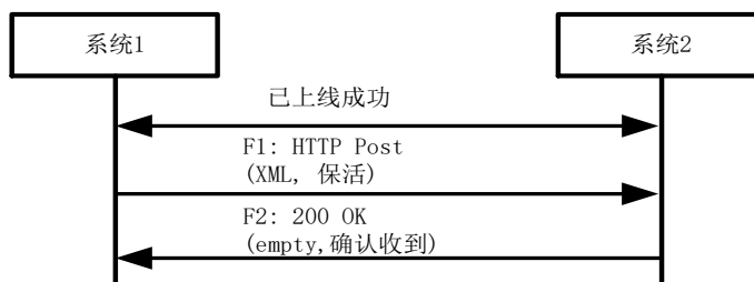
图A.2 系统心跳通知流程
