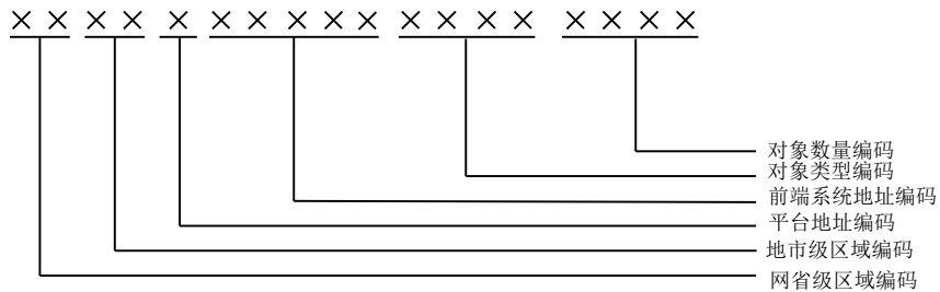
图 D.1 对象地址编码结构
