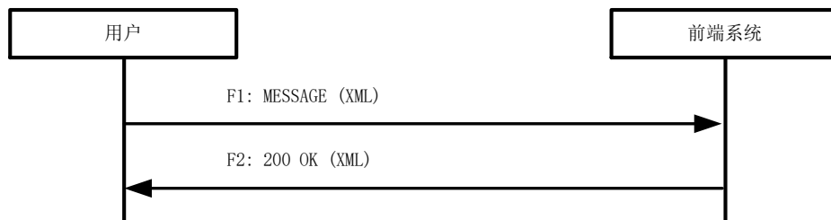
图C.6 录像检索接口流程
