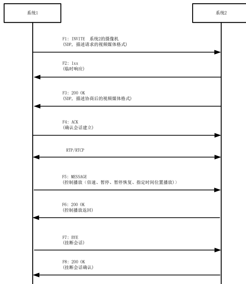
图C.10 录像回放接口流程
