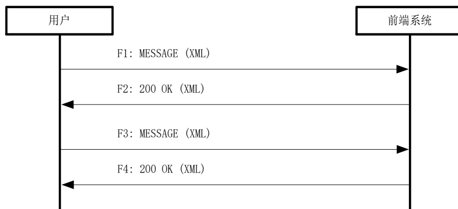
图C.20 录像计划获取及配置流程
