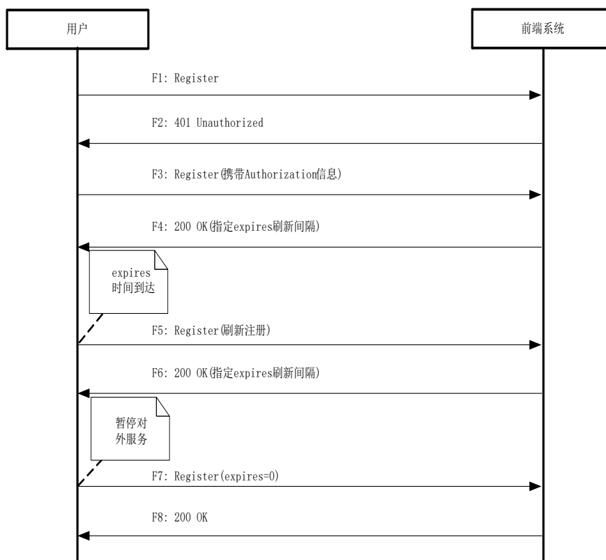
图C.1 设备登陆、登出及保活接口流程
