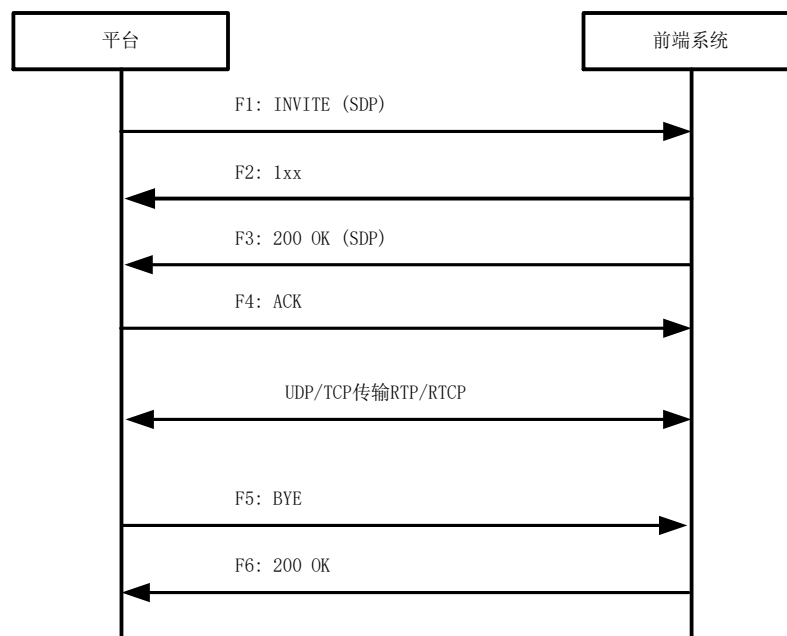
图B.7 语音对讲和广播接口流程
