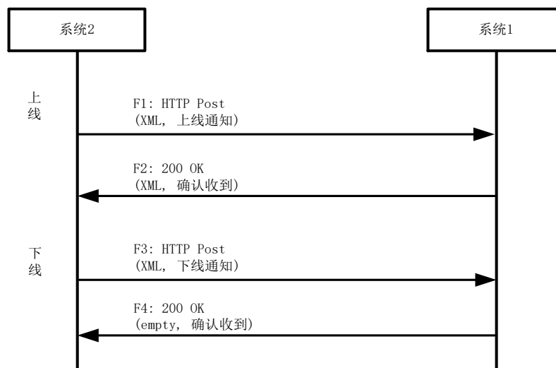
图A.1 系统上下线通知流程
