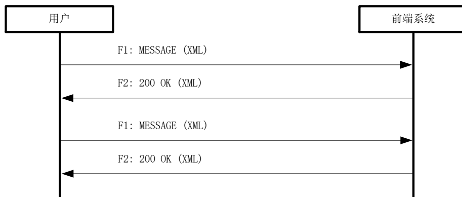
图C.24 设备时间获取及配置接口流程
