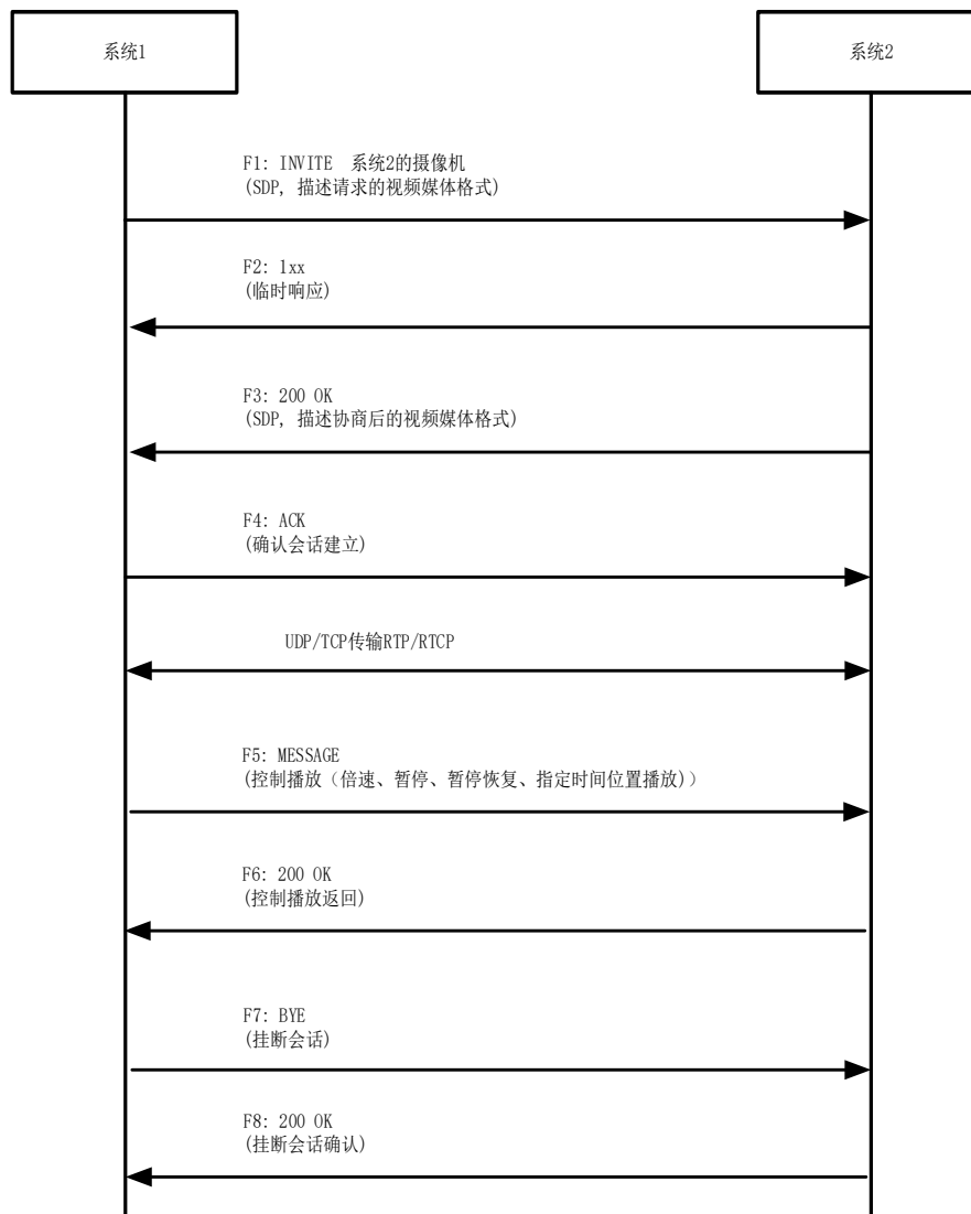
图B.11 录像回放接口流程
