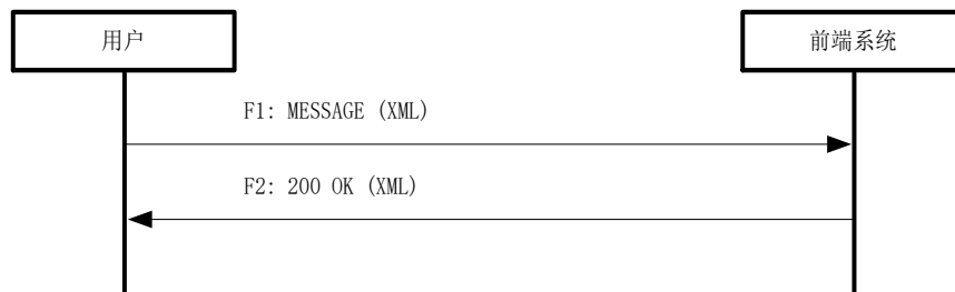
图C.3 基本信息获取流程
