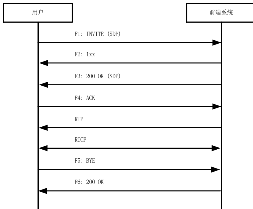
图C.7 调阅实时视频接口流程
