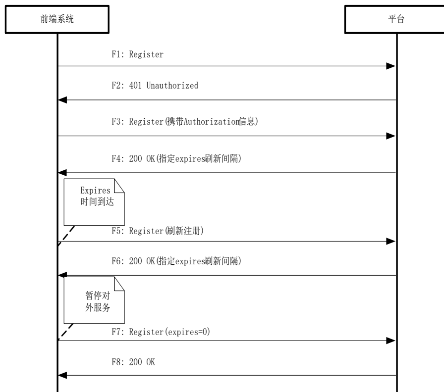
图B.1 注册接口流程
