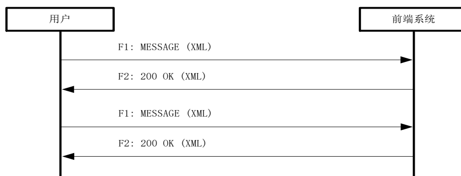
图C. 23 网络参数获取及配置流程
