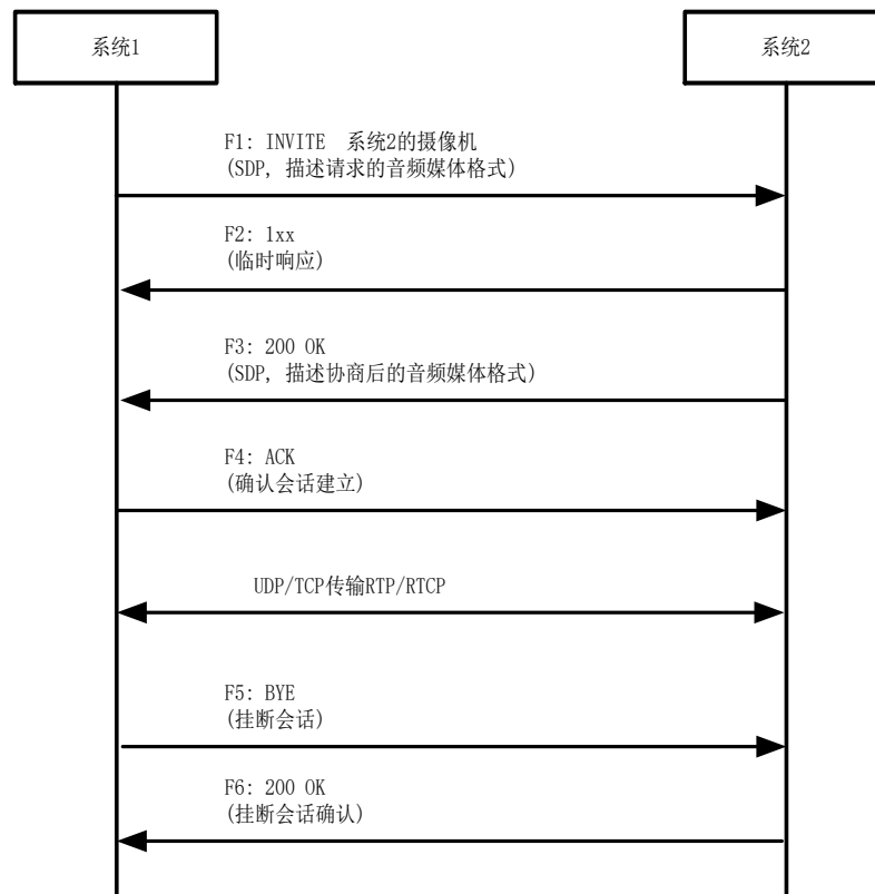
图A. 8 语音对讲和广播接口流程
