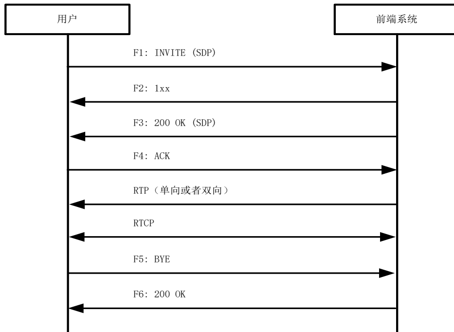
图C.8 语音对讲和广播接口流程
