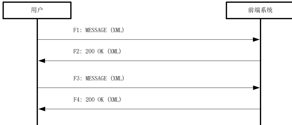
图C. 16 设备连接参数获取及配置接口流程
