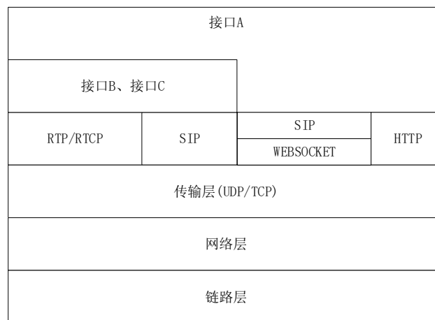
图5 接口协议结构图
