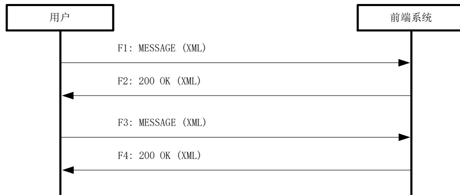
图C.19 OSD 参数获取及配置流程
