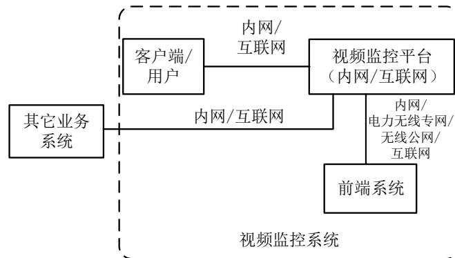
图3 视频监控平台网络连接示意图
