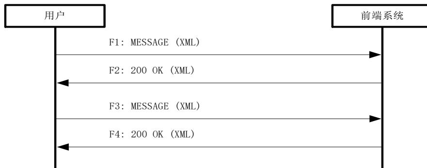
图C.18 云镜参数获取及配置流程
