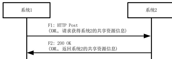
图A.3 资源信息获取接口流程
