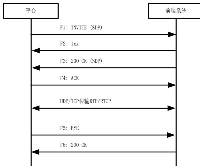
图B.6 调阅实时视频接口流程
