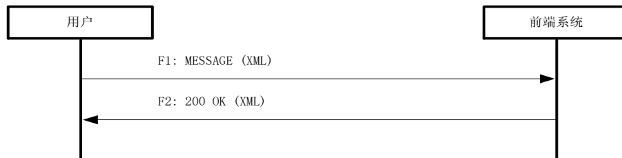
图C.14 日志信息获取流程
