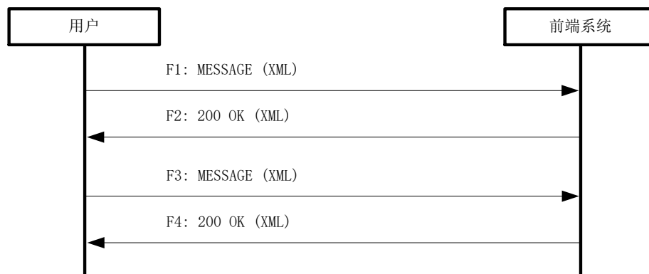
图C.21 移动侦测获取及配置流程
